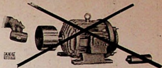
Fig. 6. Riemschijf opzetten (verkeerde methode)
