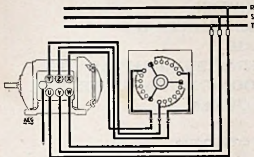
Fig. 4. Motor met statorweerstand met 3 klemmen.
